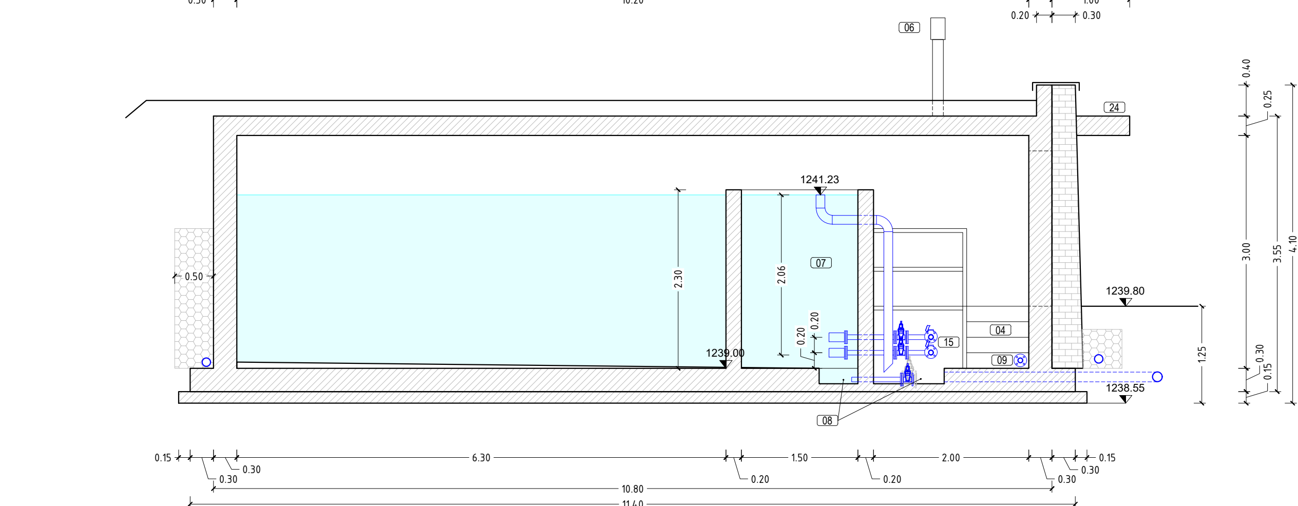
SEZ. A-A' SCALA 1:50
