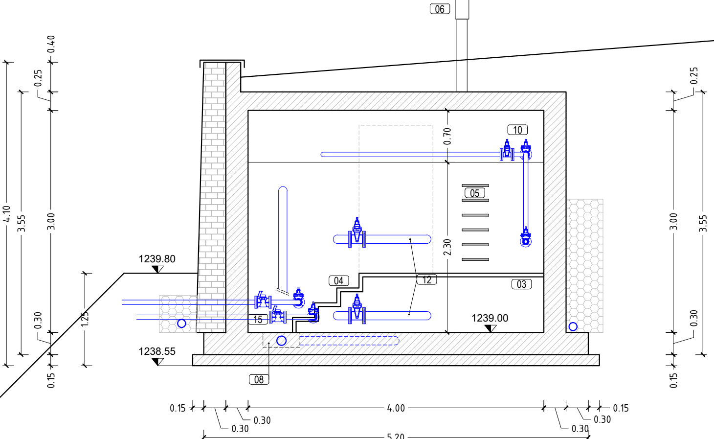
SEZ. C-C' SCALA 1:50
