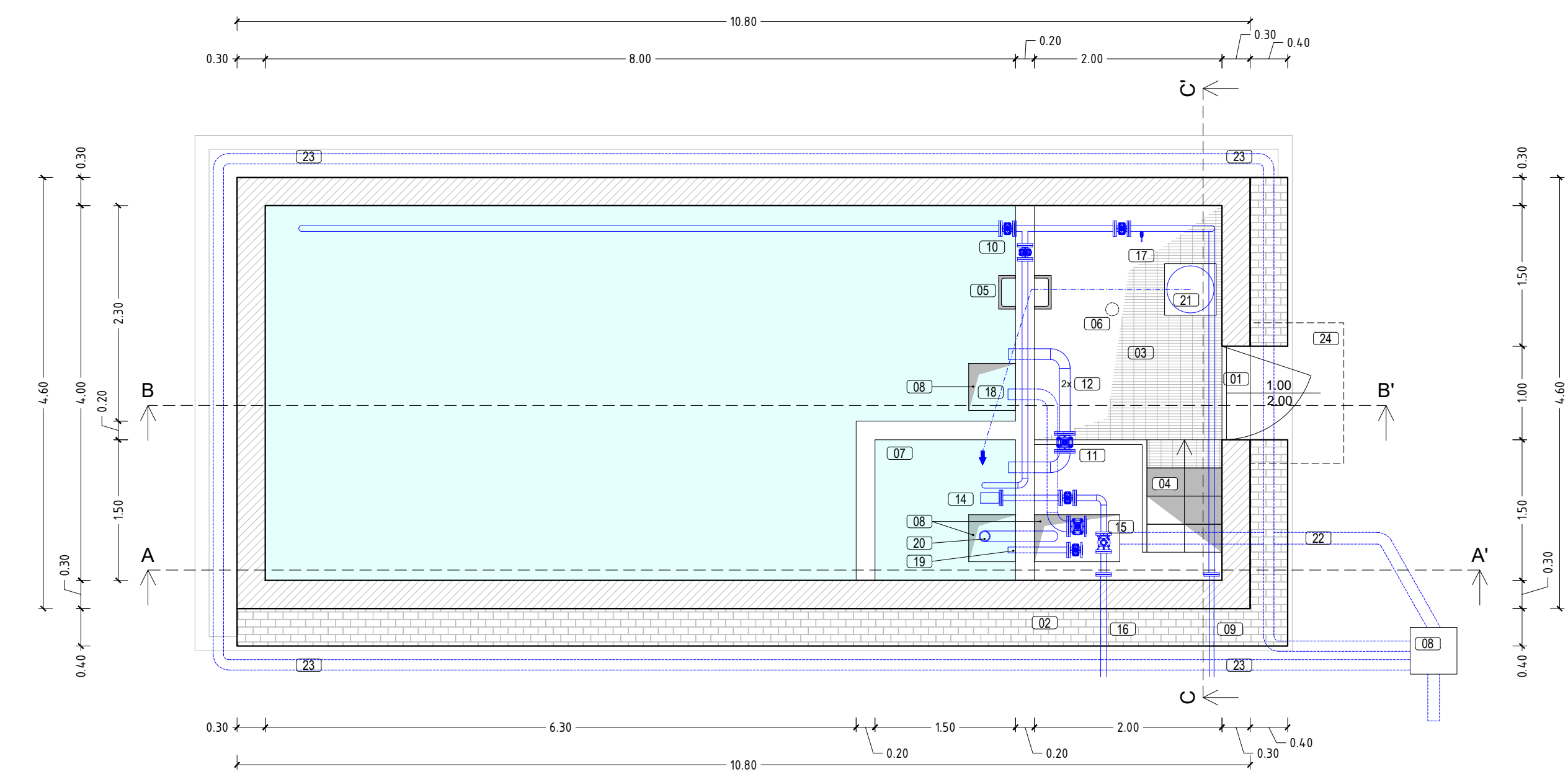
PIANTA SCALA 1:50
